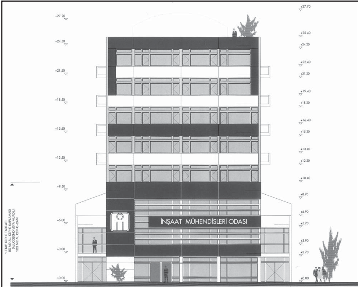
Ön Cephe
