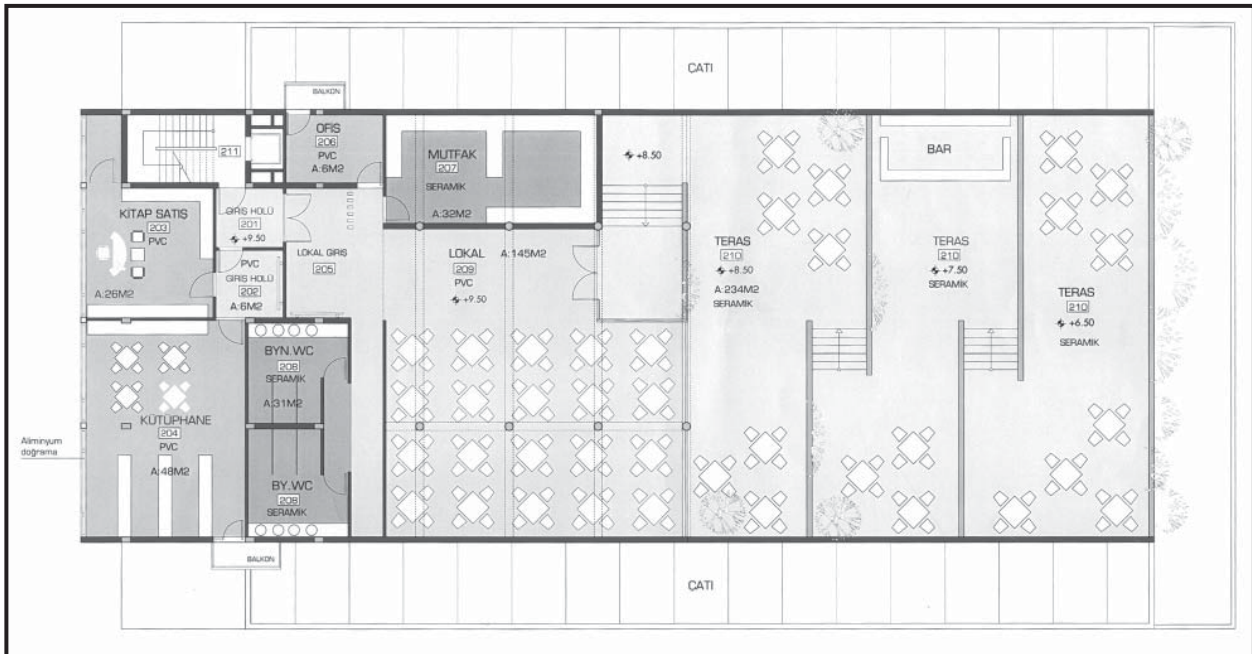
2. Kat Planı
