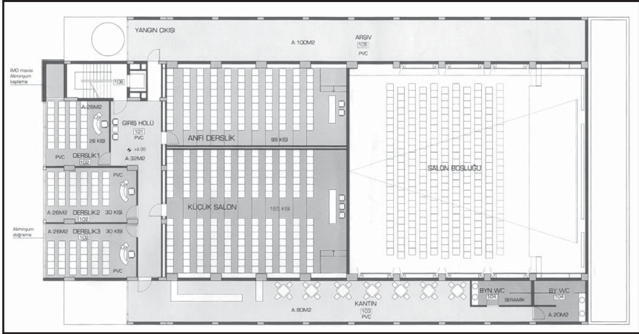
1. Kat Planı
